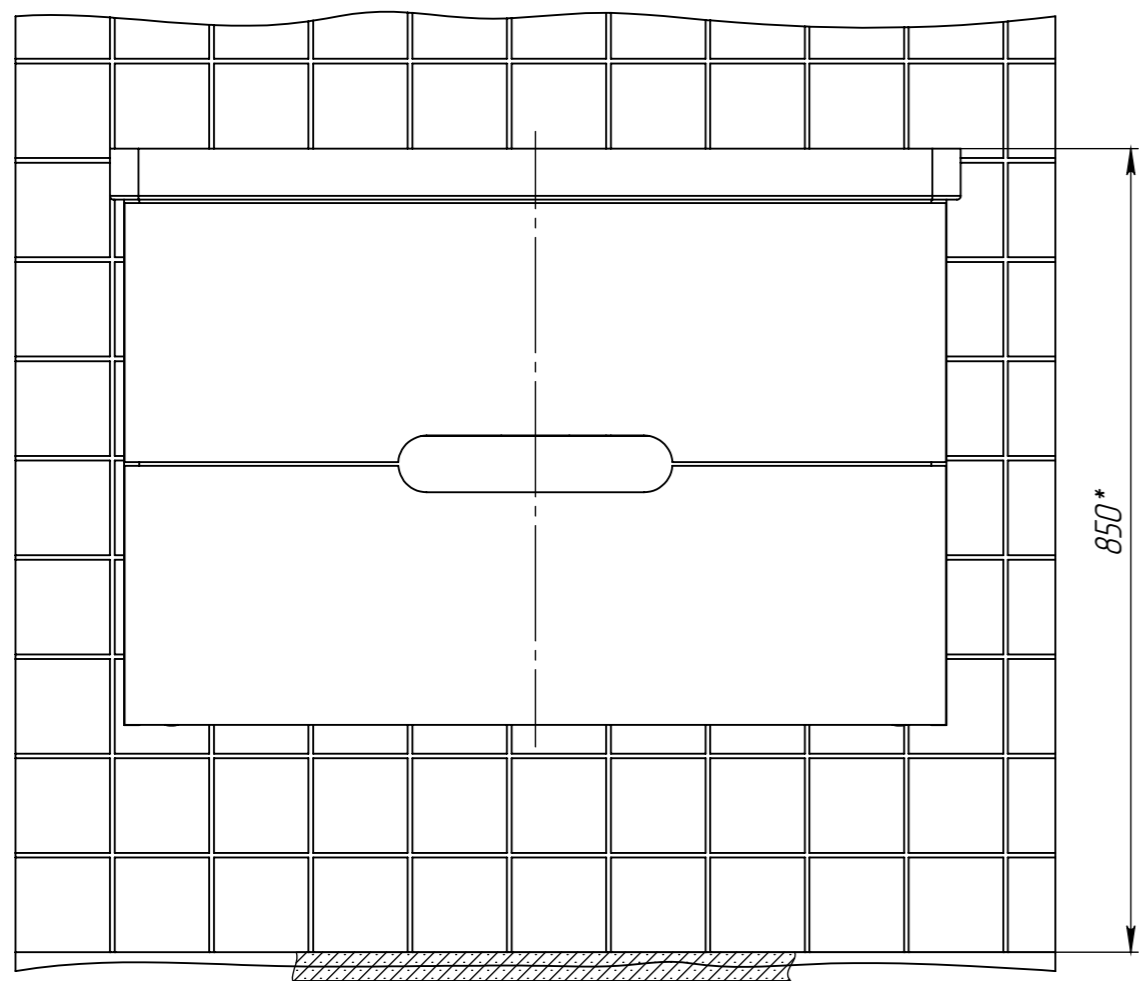
Уровень пола
